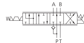
Kaldırma B Portunda Raise on B port
