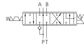
Kaldırma A Portunda Raise on A port
